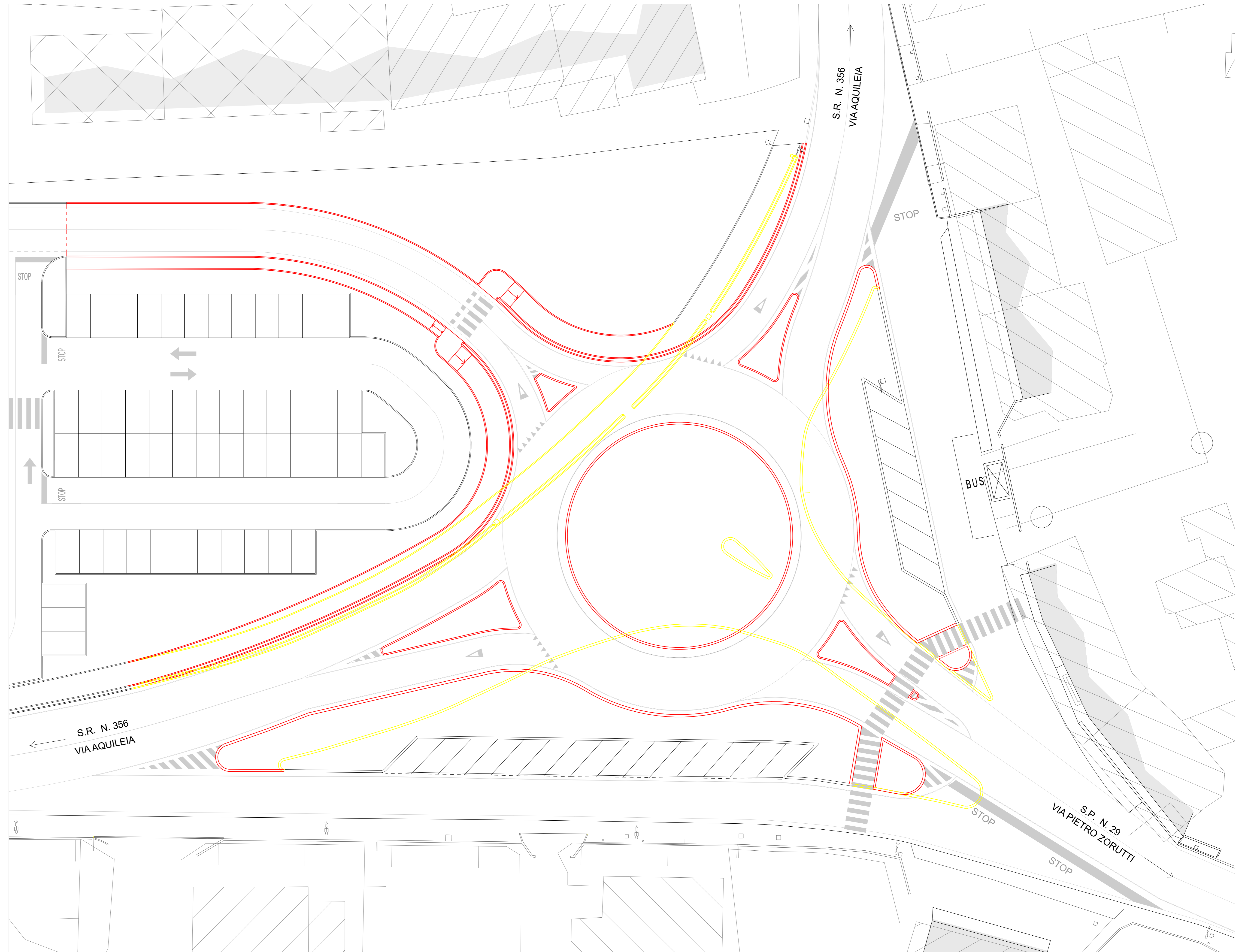
PLANIMETRIA OPERE URBANIZZAZIONE ALL'INTERNO E ALL'ESTERNO DEL P.A.C DEMOLIZIONI - COSTRUZIONI SCALA 1:200
