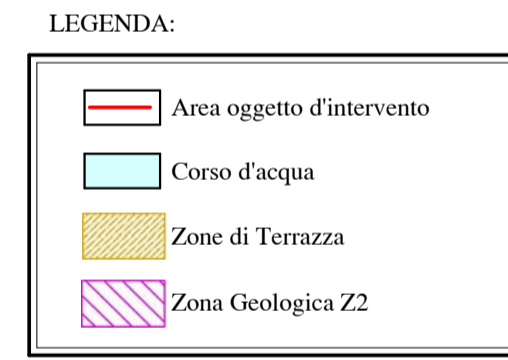
Estratto della Carta Geologica
